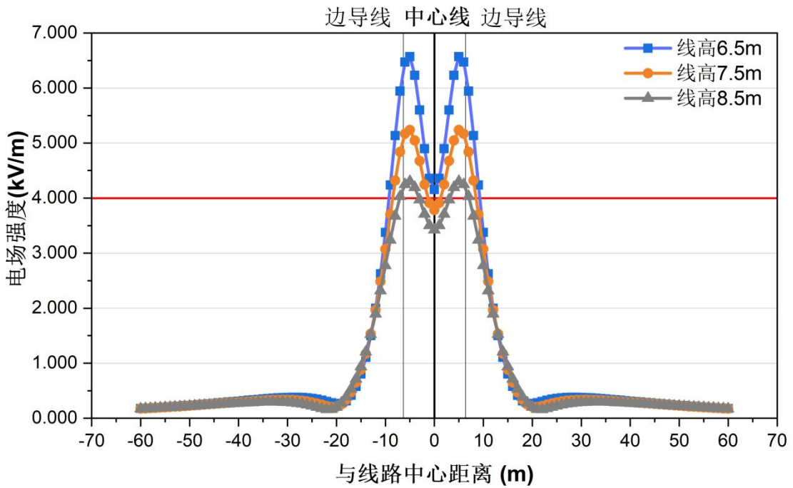
图 6.1-16a 220kV 慈柳一、二线同塔双回路迁改线路地面 1.5m 处工频电场强度变化趋势
