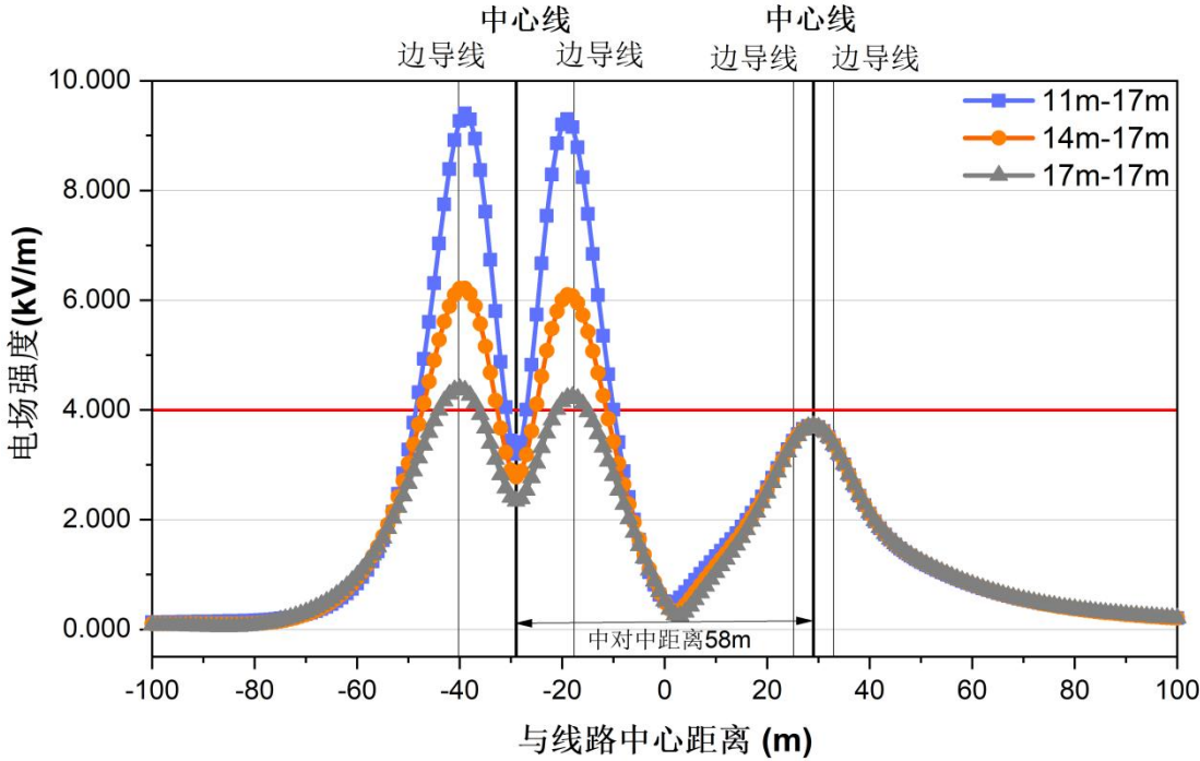
图 6.1-9a 本工程 500kV 输电线路与 500kV 源霸一线并行段地面（1.5m）工频电场强度变化趋势
