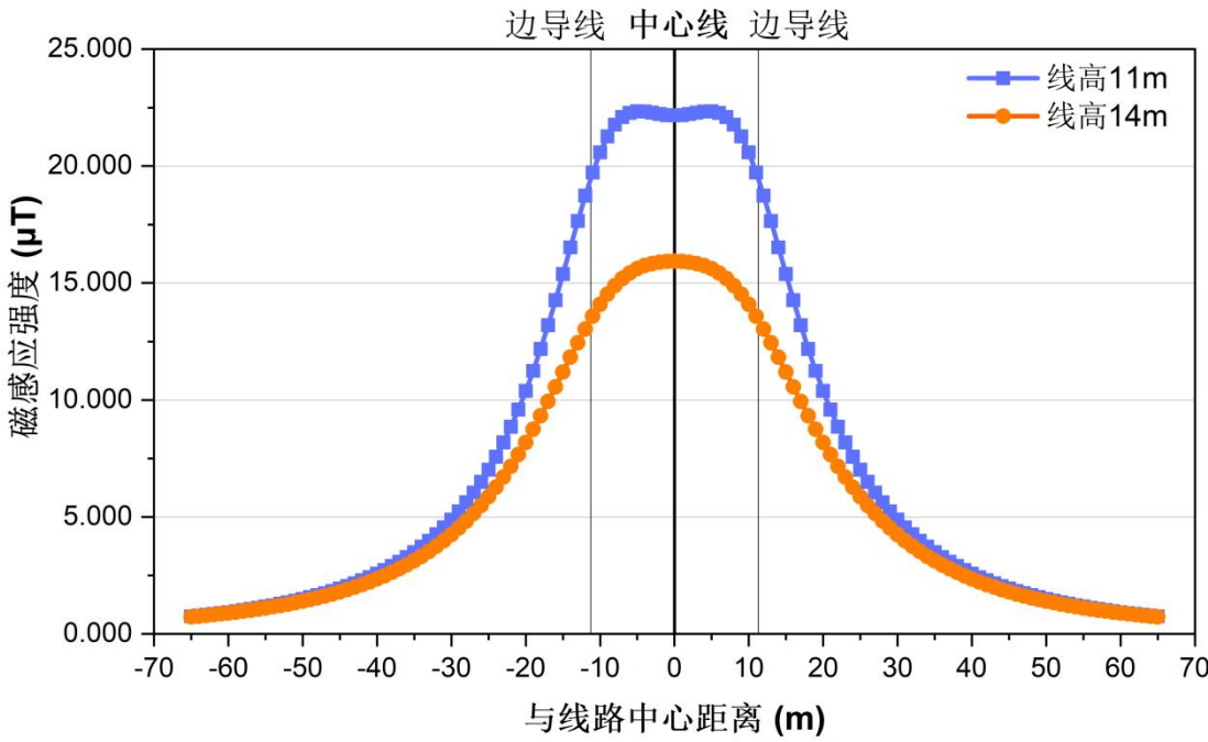
图 6.1-13b 500kV 定固一、二线同塔双回路迁改线路地面 1.5m 处工频磁感应强度变化趋势
