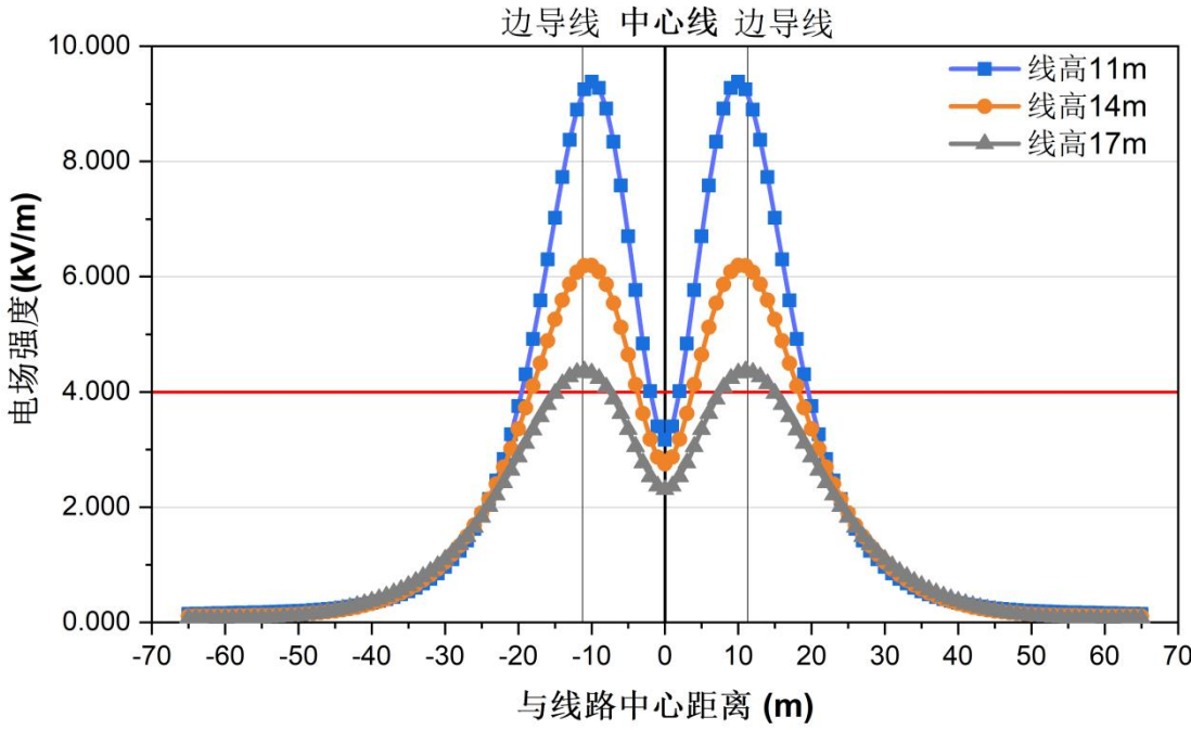
图 6.1-13a 500kV 定固一、二线同塔双回路迁改线路地面 1.5m 处工频电场强度变化趋势
