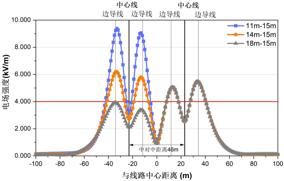
图 6.1-8a 本工程 500kV 输电线路与 500kV 定固一、二线并行段地面（1.5m）工频电场强度变化趋势
