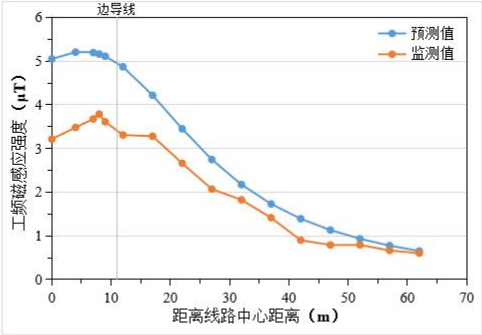
图 6.1-7 工频磁感应强度理论计算结果与实测结果对比图
