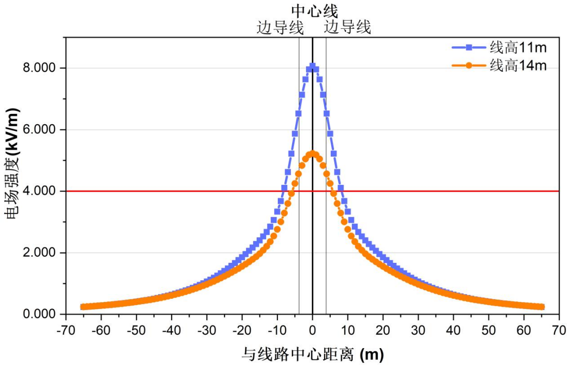
图 6.1-14a 500kV 源霸一线单回路迁改线路地面 1.5m 处工频电场强度变化趋势
