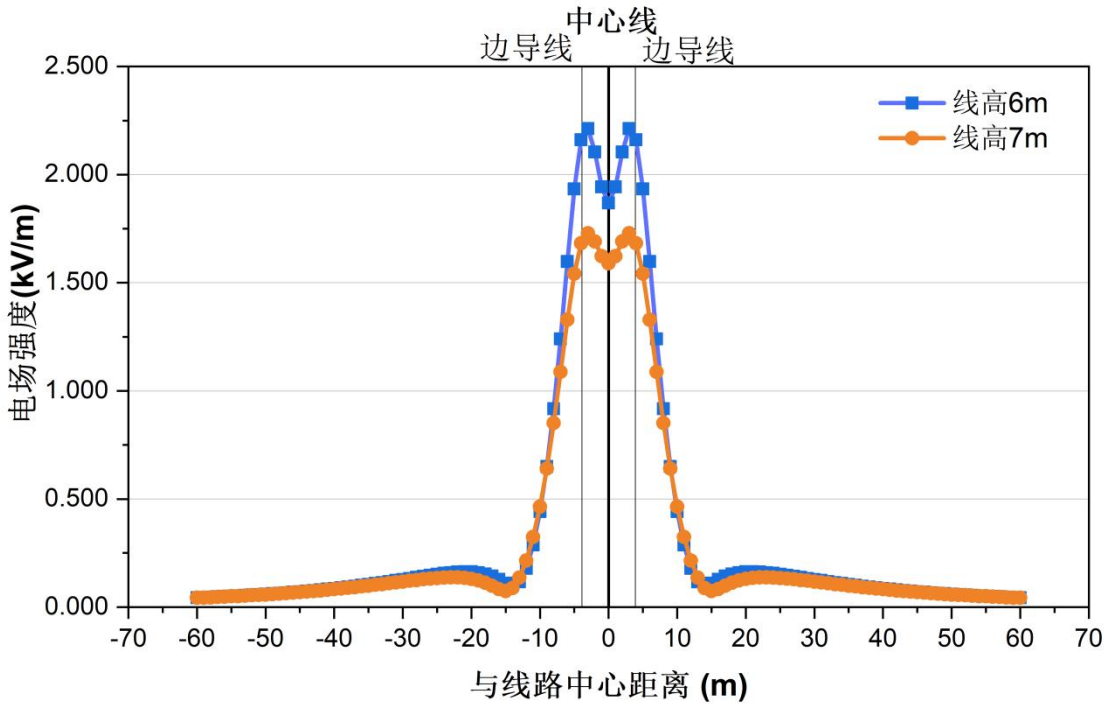
图 6.1-17a 110kV 大求一、二线同塔双回路迁改线路地面 1.5m 处工频电场强度变化趋势
