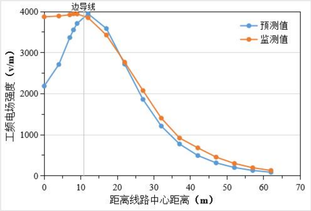
图 6.1-6 工频电场强度理论计算结果与实测结果对比图
