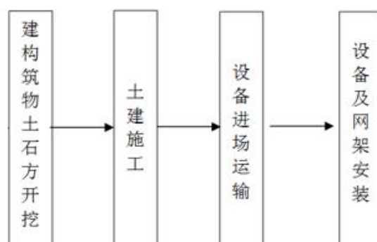
图 3.3-1 变电站工程主要施工工艺和方法
