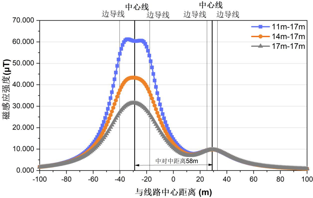
图 6.1-9b 本工程 500kV 输电线路与 500kV 源霸一线并行段地面（1.5m）工频磁感应强度变化趋势
