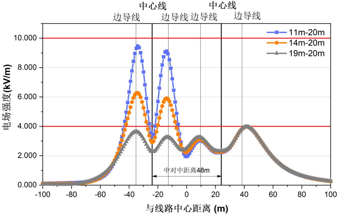
图 6.1-10a 本工程 500kV 输电线路与 500kV 源安一线并行段地面（1.5m）工频电场强度变化趋势
