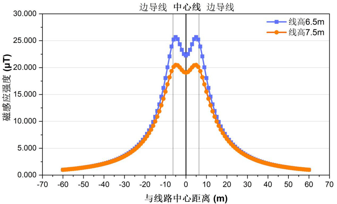
图 6.1-16b 220kV 慈柳一、二线同塔双回路迁改线路地面 1.5m 处工频磁感应强度变化趋势
