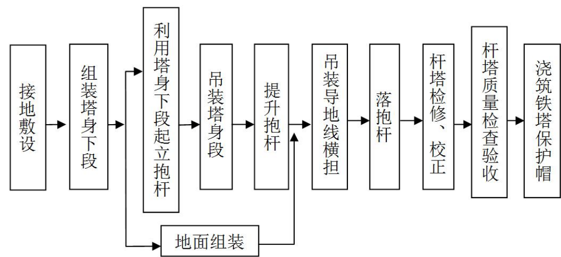
图 3.3-2 输电线路铁塔组立施工流程图
