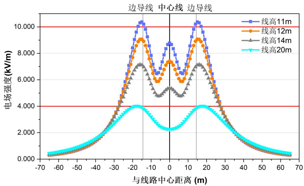
图 6.1-15a 500kV 源安一线单回路迁改线路地面 1.5m 处工频电场强度变化趋势
