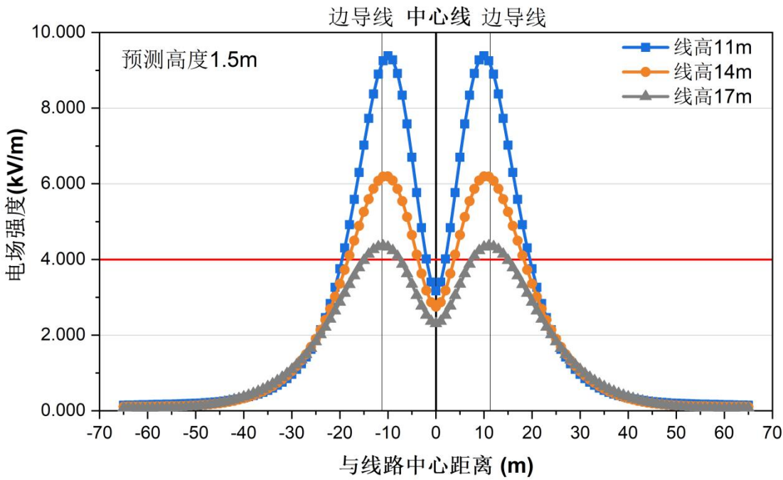
图 6.1-4a 同塔双回路 500-MC21S-ZK 塔 1.5m 高处工频电场强度变化趋势
