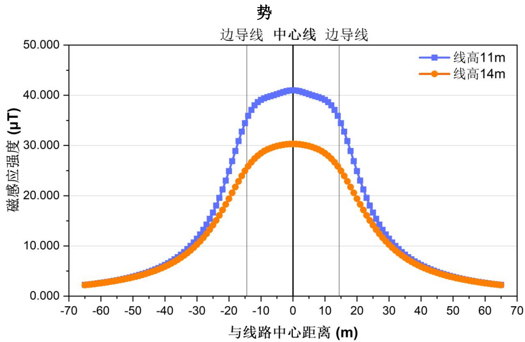
图 6.1-15b 500kV 源安一线单回路迁改线路地面 1.5m 处工频磁感应强度变化趋势
