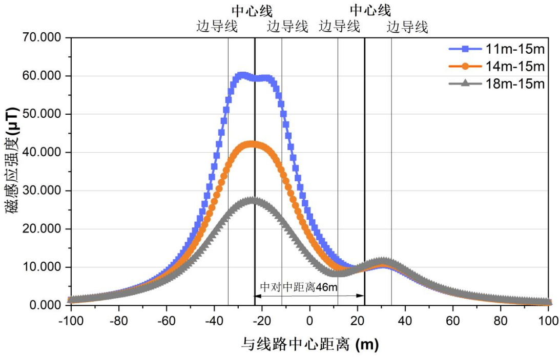
图 6.1-8b 本工程 500kV 输电线路与 500kV 定固一、二线并行段地面（1.5m）工频磁感应强度变化趋势
