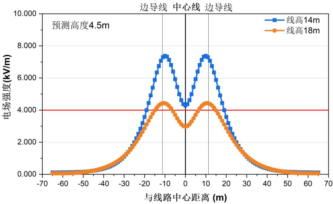
图 6.1-4b 同塔双回路 500-MC21S-ZK 塔 4.5m 高处工频电场强度变化趋势
