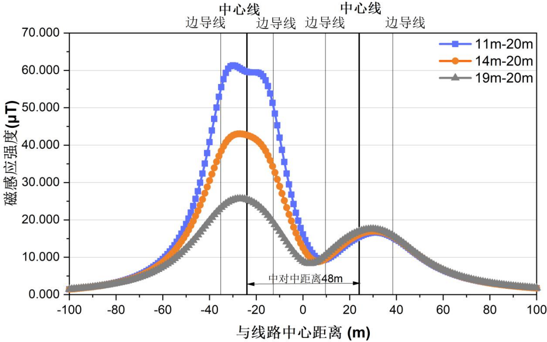
图 6.1-10b 本工程 500kV 输电线路与 500kV 源安一线并行段地面（1.5m）工频磁感应强度变化趋势
