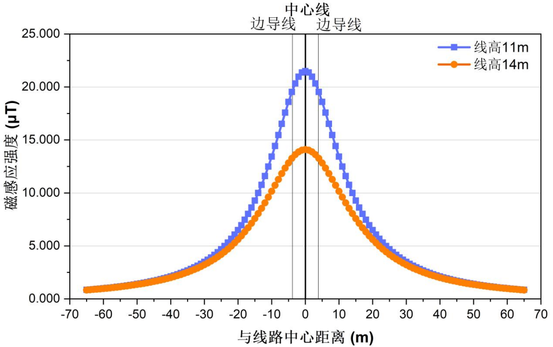
图 6.1-14b 500kV 源霸一线单回路迁改线路地面 1.5m 处工频磁感应强度变化趋势
