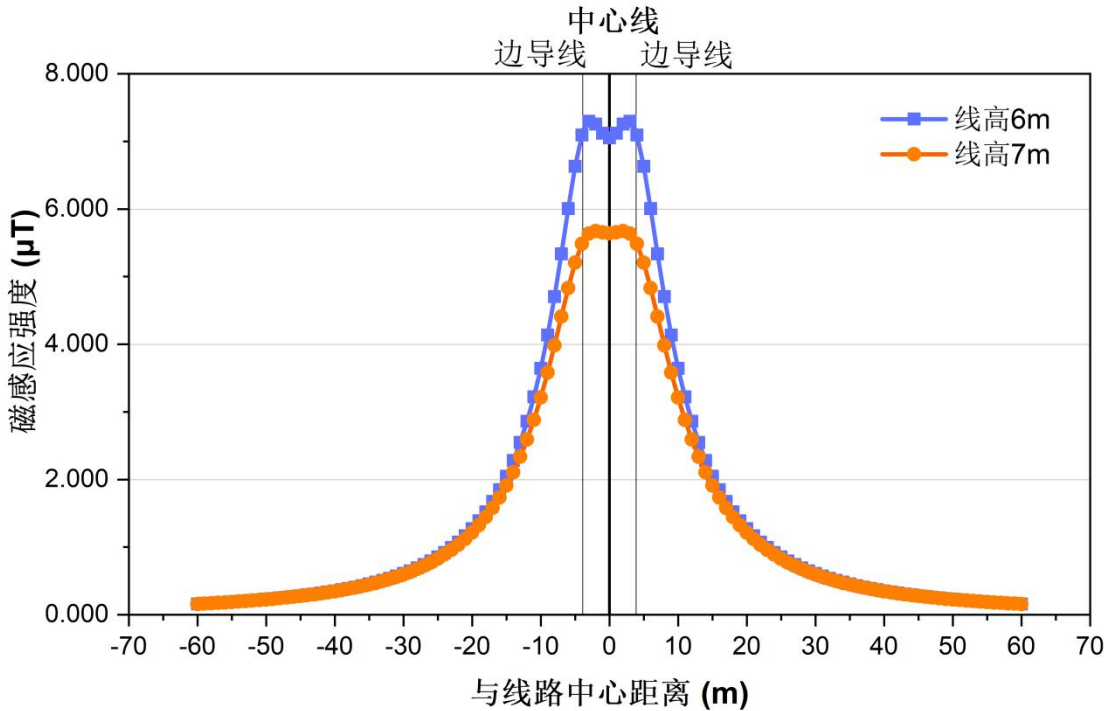
图 6.1-17b 110kV 大求一、二线同塔双回路迁改线路地面 1.5m 处工频磁感应强度变化趋势
