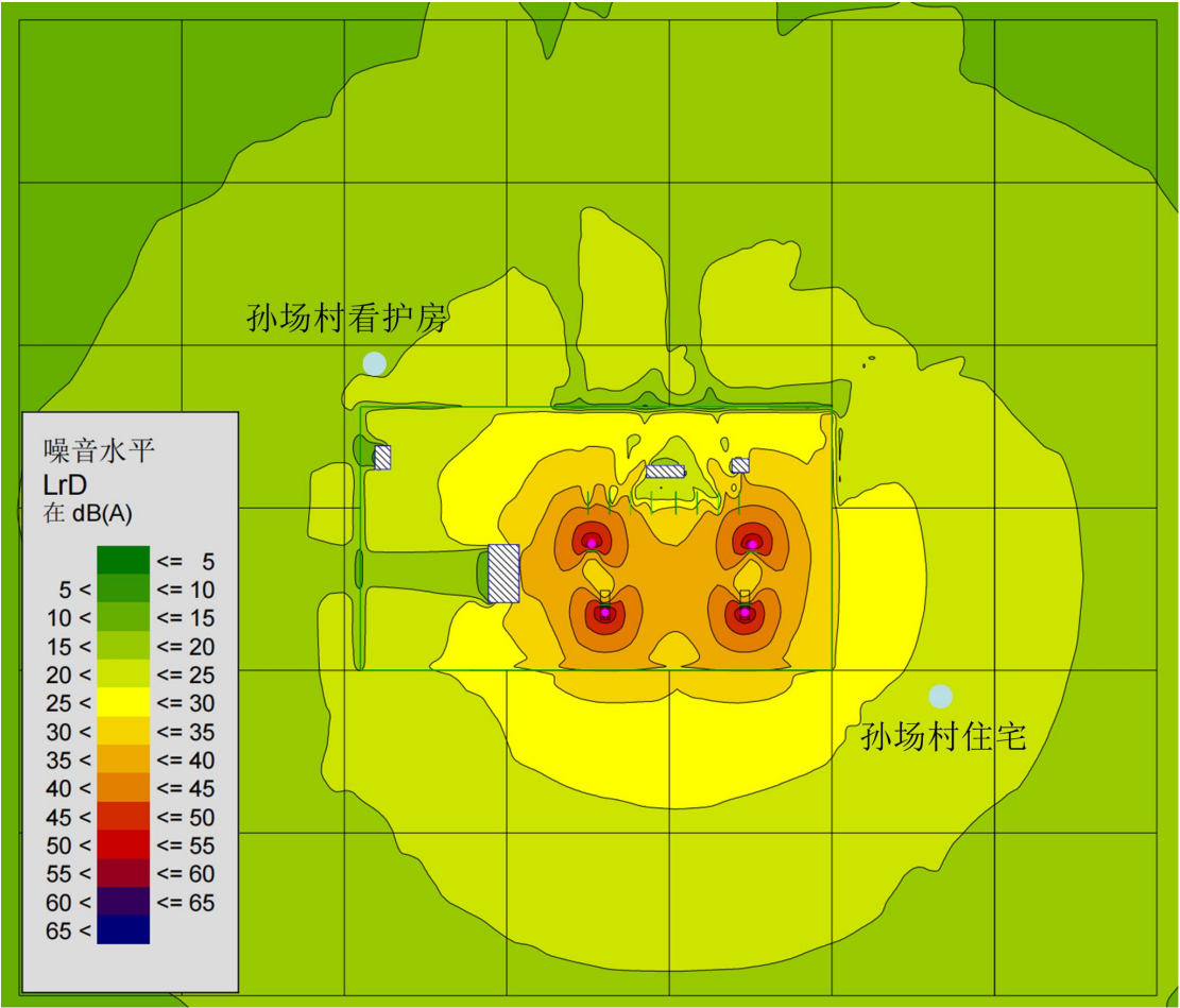
图 6.2-2 新航城 500kV 变电站噪声贡献值等声级曲线预测图
