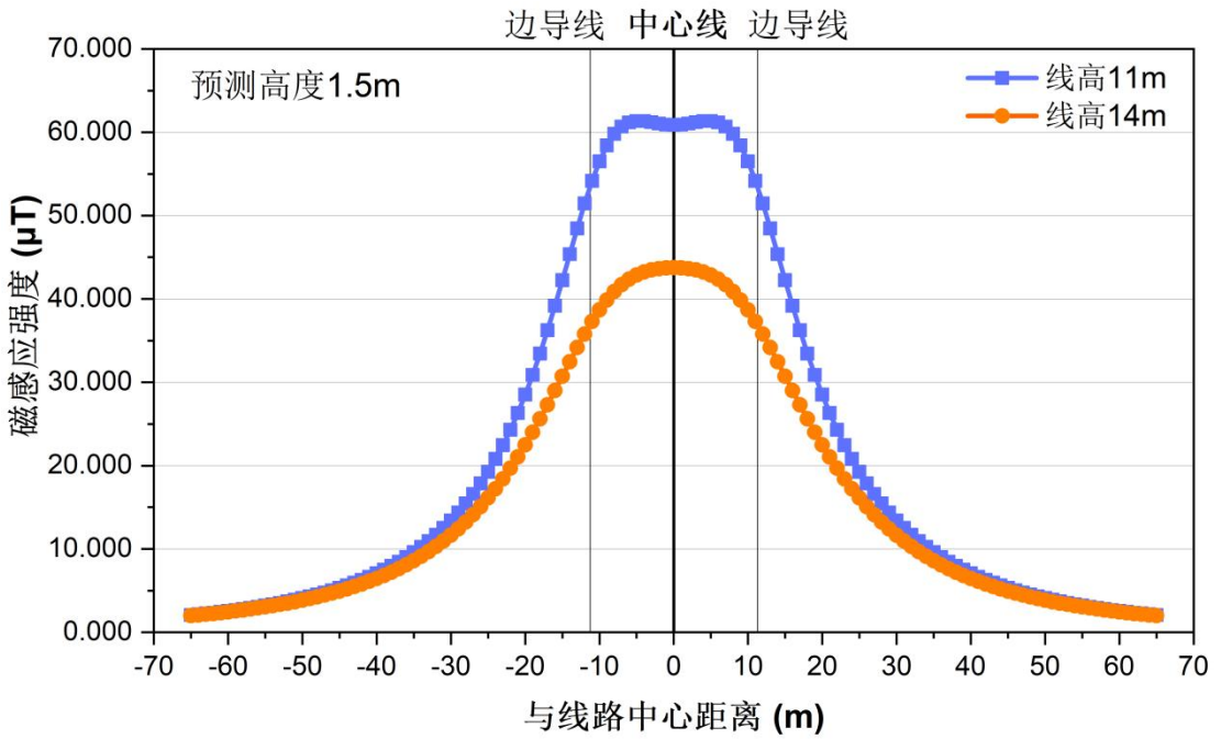
图 6.1-5a 同塔双回路 500-MC21S-ZK 塔地面（1.5m）工频磁感应强度变化趋势
