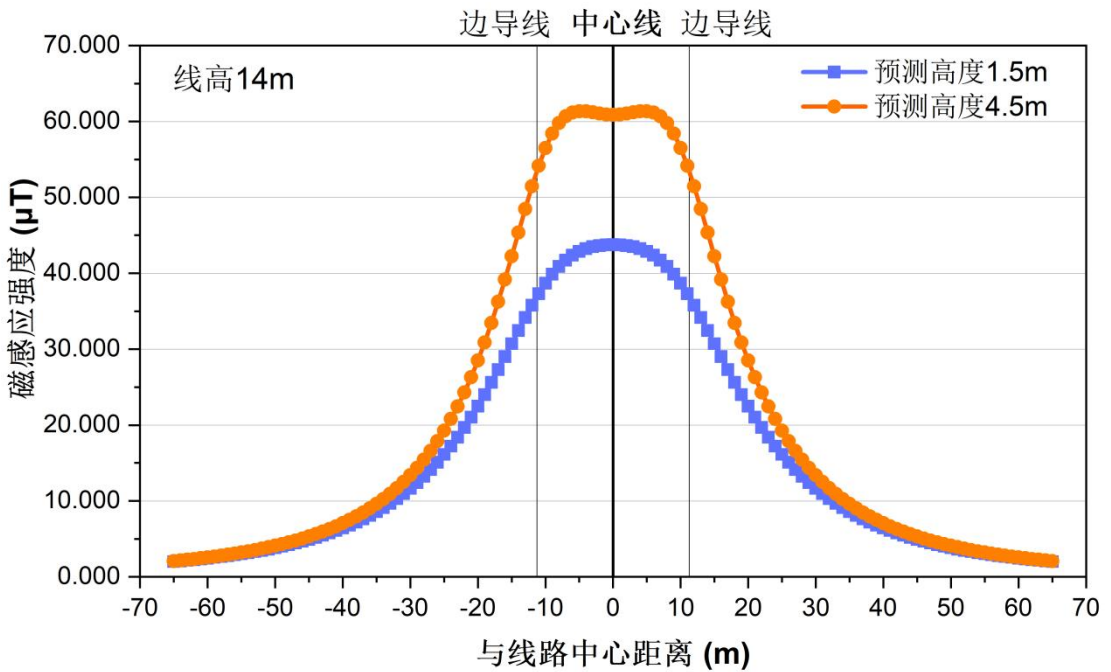
图 6.1-5b 同塔双回路 500-MC21S-ZK 塔线高 14m 时不同预测高度工频磁感应强度变化趋势
